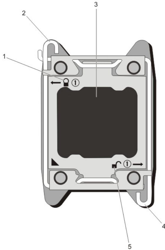
그림 35. 프로세서 실드 레버 열기 및 닫기 시퀀스
