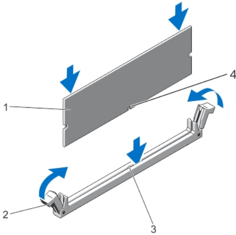
그림 13. 메모리 모듈 장착
