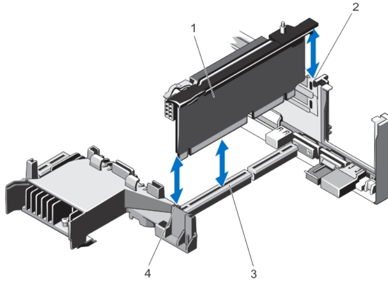
그림 28. 확장 카드 라이저 2 분리 및 설치
