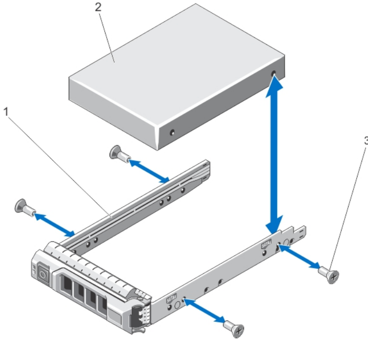
그림 17. 하드 드라이브 캐리어에서 하드 드라이브 분리 및 설치
