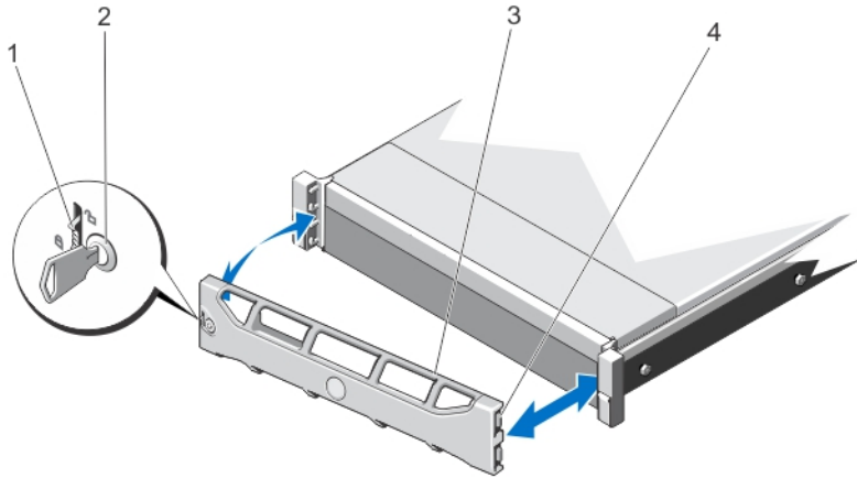
그림 7. 전면 베젤 분리 및 설치
