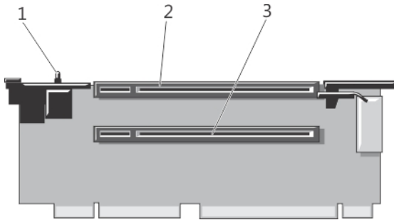
그림 29. 확장 카드 라이저 2의 커넥터 식별
