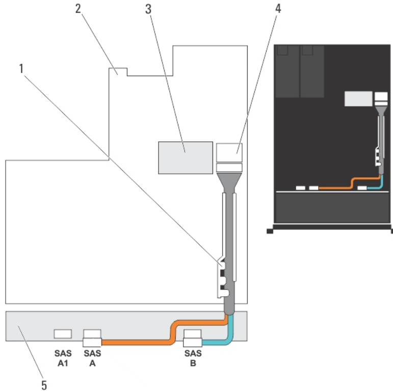
그림 41. 케이블 연결 다이어그램 – 3.5인치 (x12) SAS 후면판
