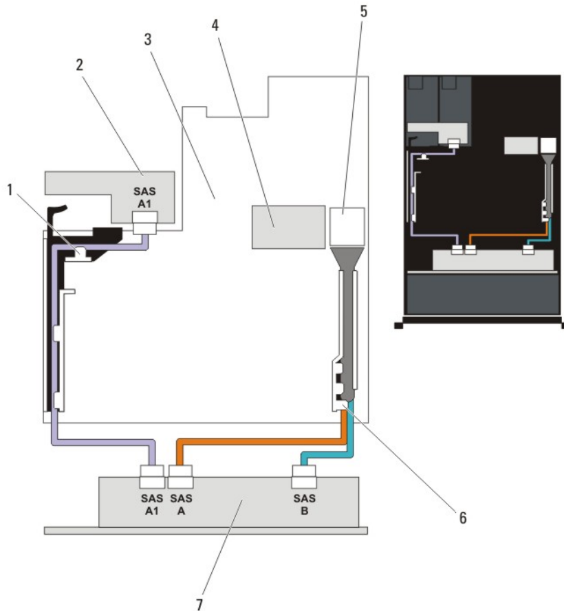
그림 43. 케이블 연결 다이어그램—선택 사양 2.5인치 (x2) 하드 드라이브 후면판(후면)
