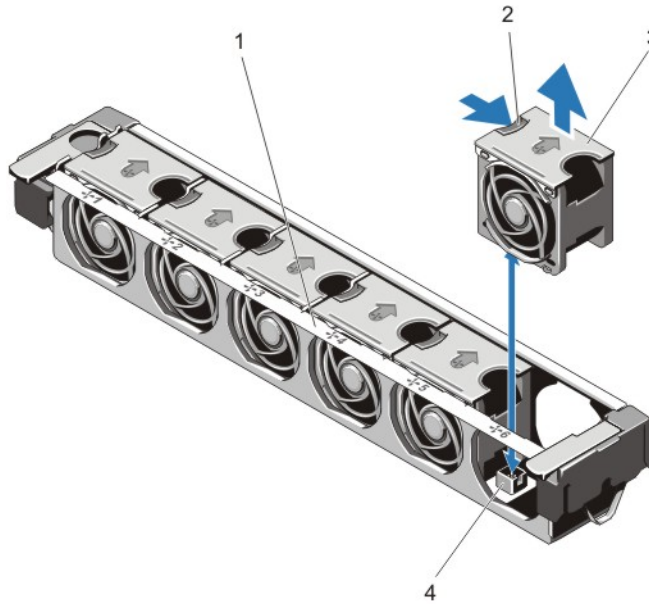
그림 18. 냉각 팬 분리 및 설치
