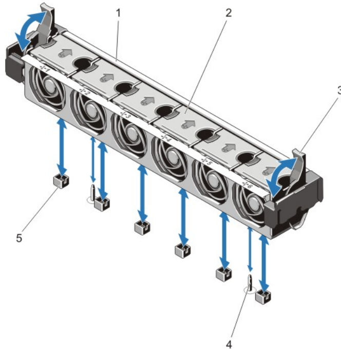
그림 19. 냉각 팬 조립품 분리 및 설치
