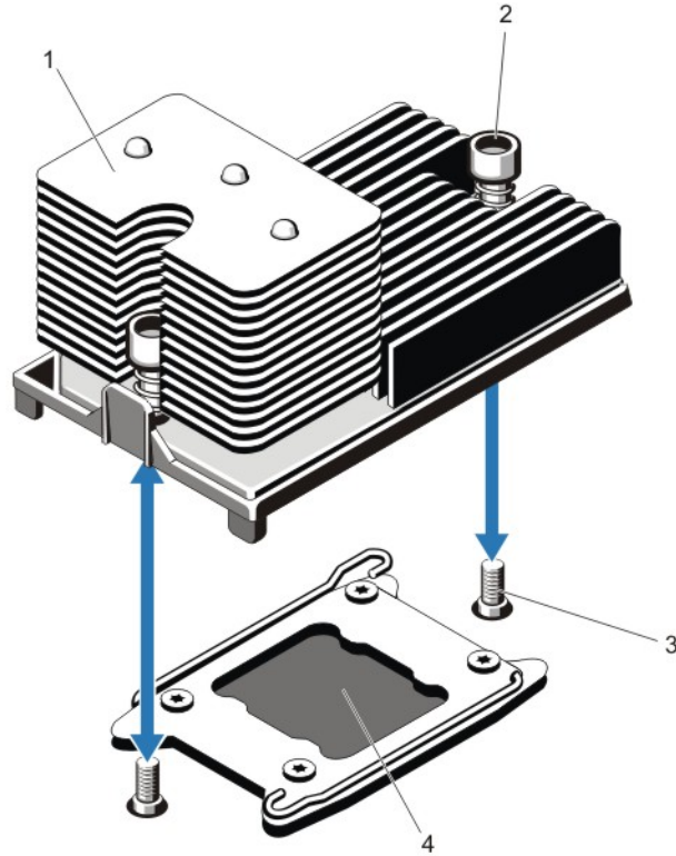
그림 34 . 프로세서 방열판 분리 및 설치
