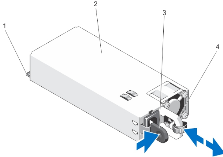
그림 37. AC 전원 공급 장치 분리 및 설치
