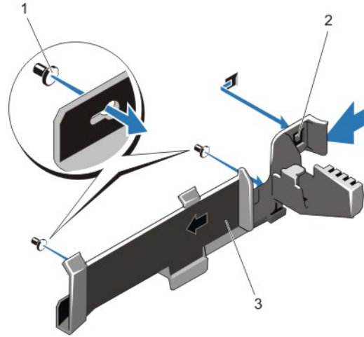
그림 23. 케이블 고정 브래킷 분리 및 설치
