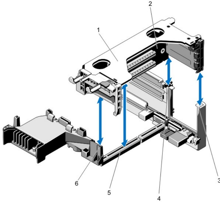
그림 26. 확장 카드 라이저 1 분리 및 설치
