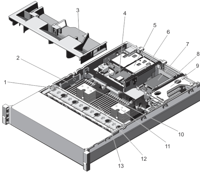
그림 6. 시스템 내부
