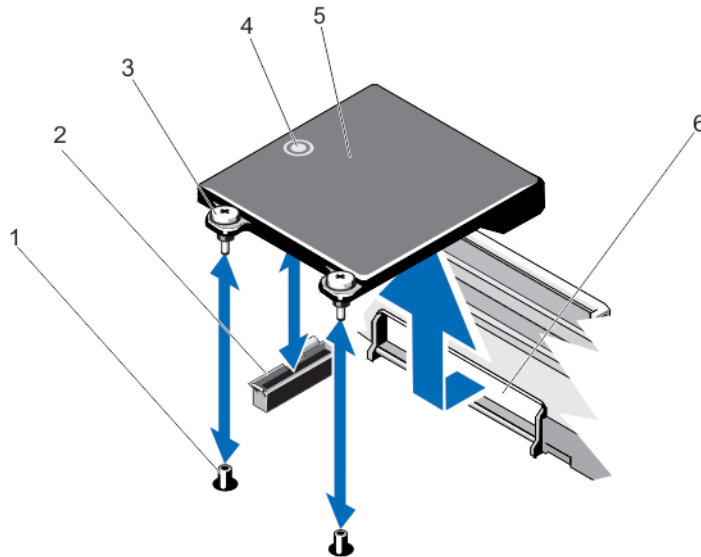
그림 33. 네트워크 도터 카드 분리 및 설치
