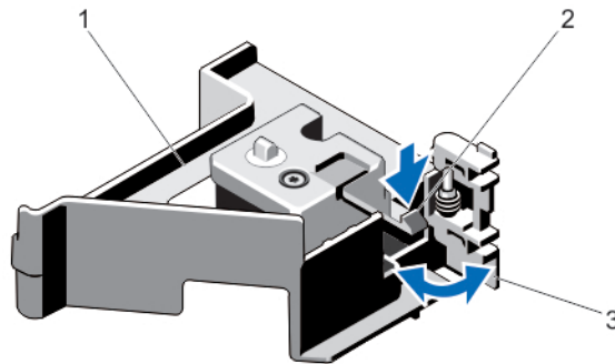
그림 22. PCIe 카드 홀더 래치 열기 및 닫기
