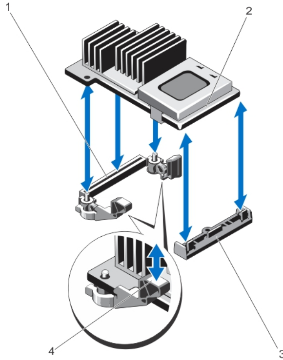
그림 32. 내장형 저장소 컨트롤러 카드 분리 및 설치
