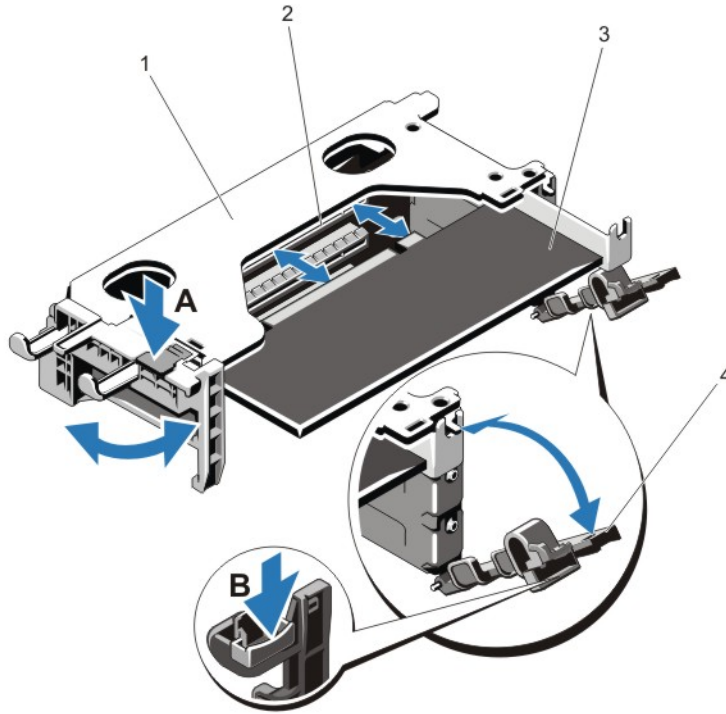
그림 25. 확장 카드 라이저 1 분리 및 설치
