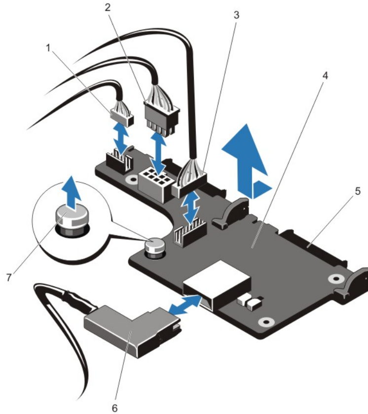
그림 42. 선택 사양 2.5인치 (x2) 하드 드라이브 후면판 분리 및 설치
